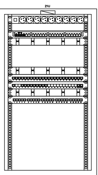
Rys. Rozmieszczenie elementów w szafie FD-0A
