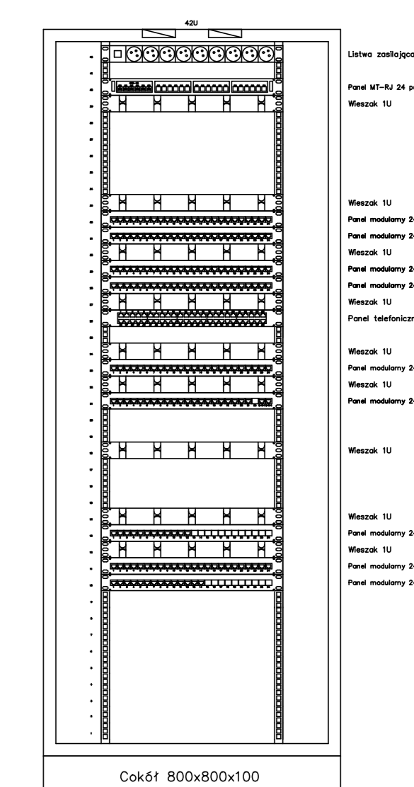
Rys. Rozmieszczenie elementów w szafie FD-1G
