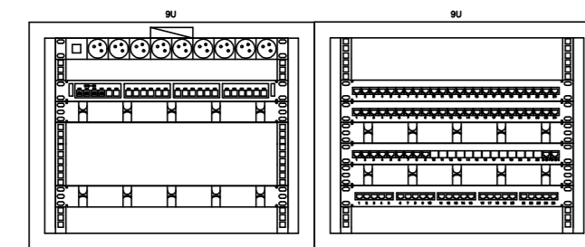
Rys. Rozmieszczenie elementów w szafie FD-0B
