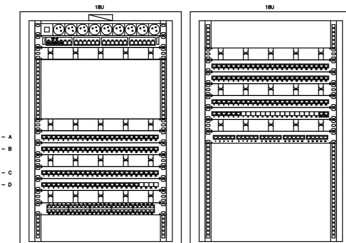
Rys. Rozmieszczenie elementów w szafie FD-2B
