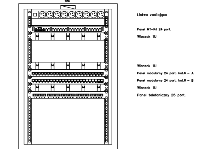
Rys. Rozmieszczenie elementów w szafie FD-0F
