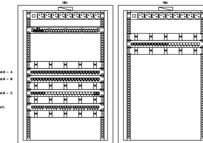
Rys. Rozmieszczenie elementów w szafie FD-1F
