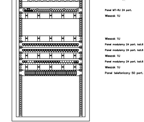
Rys. Rozmieszczenie elementów w szafie FD-0E
