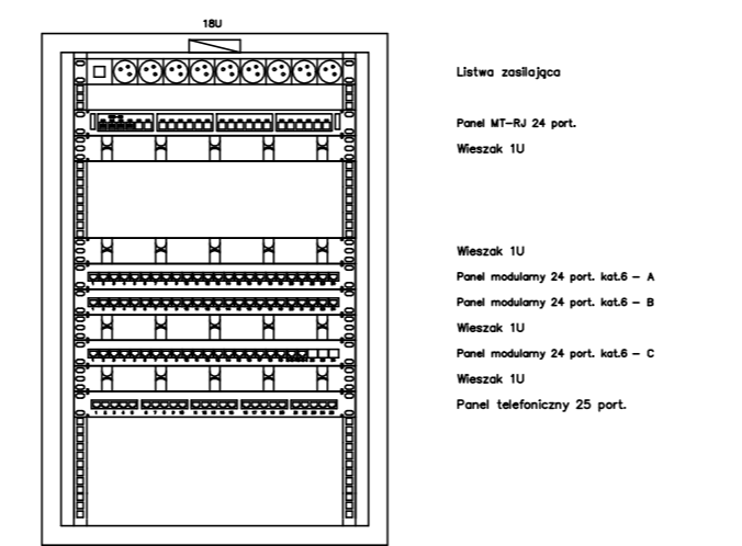
Rys. Rozmieszczenie elementów w szafie FD-0D
