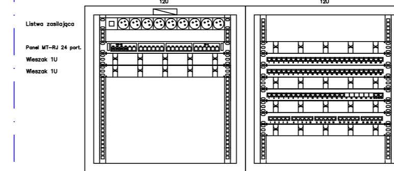
Rys. Rozmieszczenie elementów w szafie FD-0E
