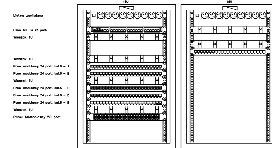
Rys. Rozmieszczenie elementów w szafie FD-0C
