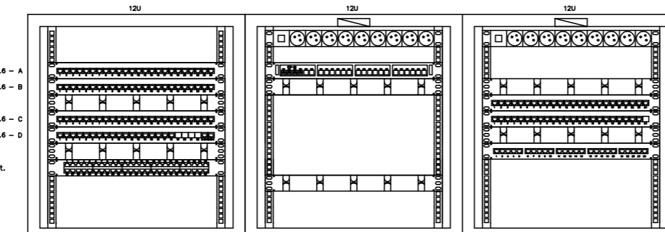
Rys. Rozmieszczenie elementów w szafie FD-2C
