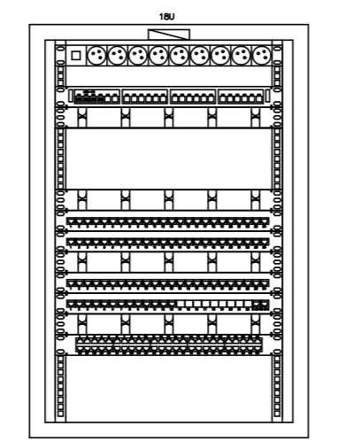
Rys. Rozmieszczenie elementów w szafie FD-0C
