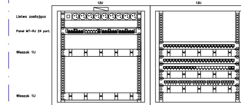
Rys. Rozmieszczenie elementów w szafie FD-1E
