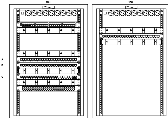
Rys. Rozmieszczenie elementów w szafie FD-1D
