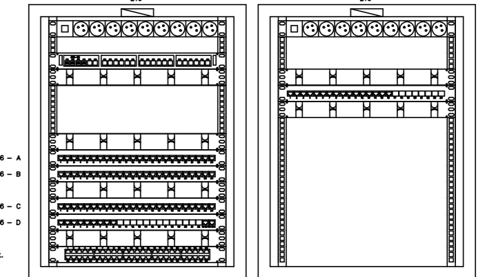
Rys. Rozmieszczenie elementów w szafie FD-0G
