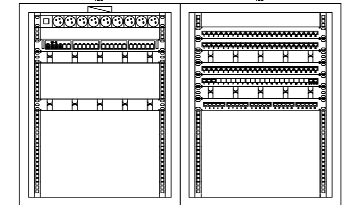
Rys. Rozmieszczenie elementów w szafie FD-0D
