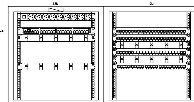
Rys. Rozmieszczenie elementów w szafie FD-2A
